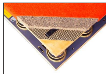
Plateau renforcé en fibre de carbone
