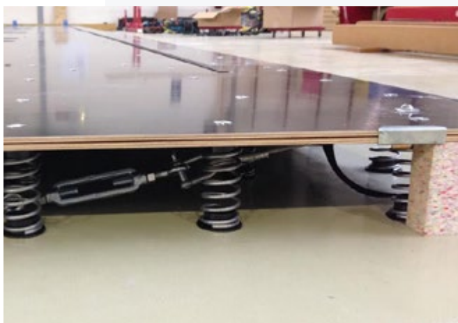
Blocage en rotation du plancher par câble d'arrêt.
